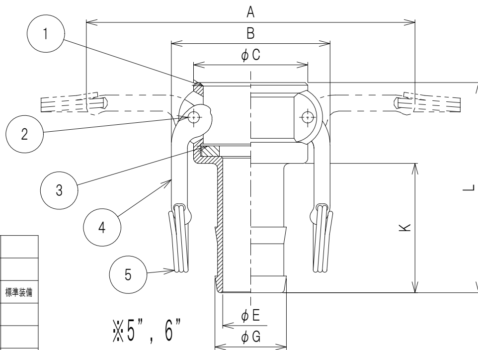
633-C SST サイズ別寸法表 (単位: mm)
